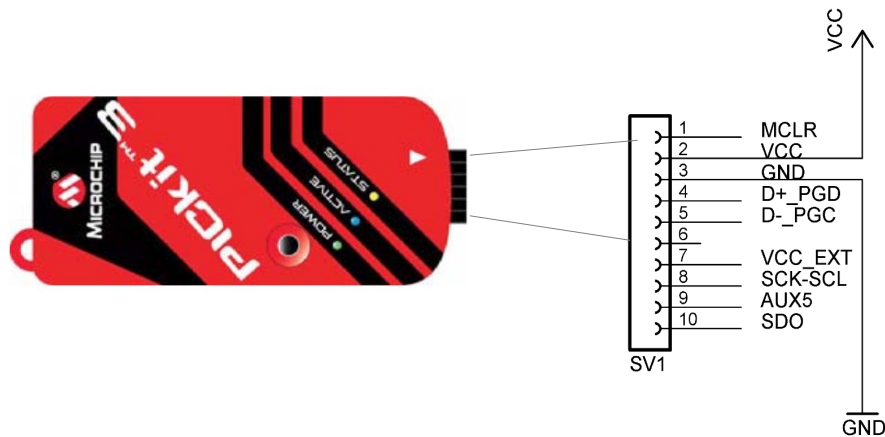
Figura 1: Connessione del programmatore PICKIT 3 alla scheda miniCOM USB.
